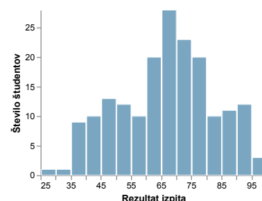
Slika 36: Histogram porazdelitve rezultatov izpita. Graf razkrije asimetrijo in morebitno večvršnost porazdelitve.
