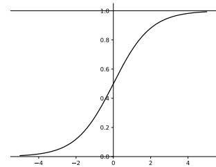
Slika 22: Sigmoidna funkcija.
