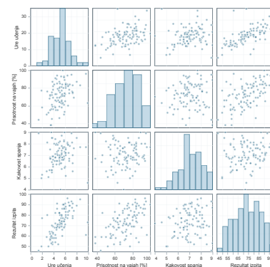
Slika 43: Matrika razsevnih diagramov prikazuje parne odnose med številom ur učenja, prisotnostjo na vajah, kakovostjo spanja in rezultatom izpita. Vsaka celica vsebuje razsewni diagram za določen par spremenljivk, diagonala pa prikazuje porazdelitve posameznih spremenljivk. Vidna je pozitivna povezava med časom učenja in rezultatom izpita ter šibkejša povezanost drugih dejavnikov.
