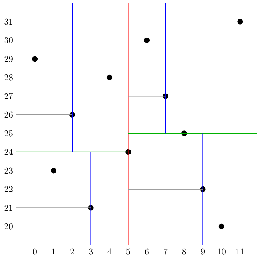
Slika 2: Množica točk in njena razdelitev glede na KD-drevo na sliki 3. Rdeča daljica pripada globini 0, zeleni pripadajo globini 1, modre pripadajo globini 2, sive pa globini 3. Točke na navpičnih daljicah pripadajo levim odsekom, točke na vodoravnih pa spodnjim odsekom.
