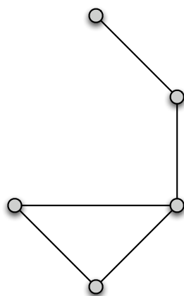
H_1 \subseteq G
