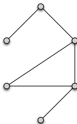
H_2 \subseteq G , vpjet.
