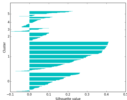
„eksterci“ (K=6)
