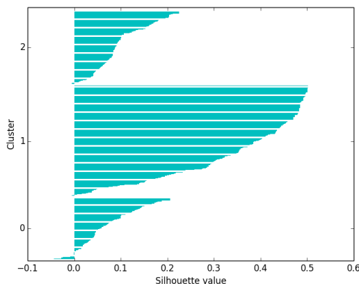
„eksterci“ (K=3)
