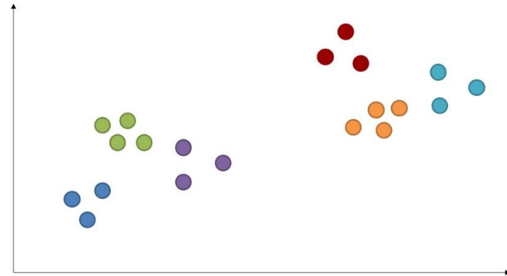
6 skupin
